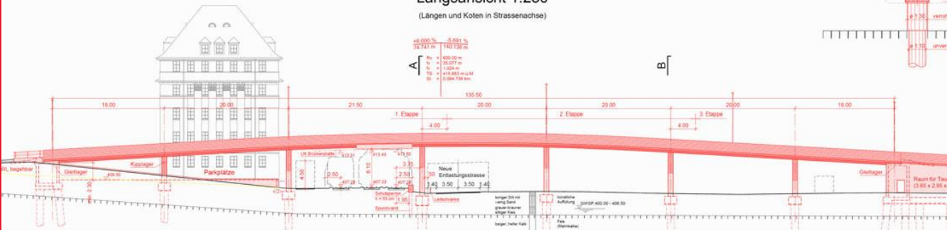
Längsansicht 1:250 (Längen und Koten in Strassenachse)
